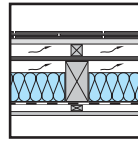
Steildach mit Wärmedämmschicht zwischen dem Tragwerk – Zweifach belüftetes Dach
